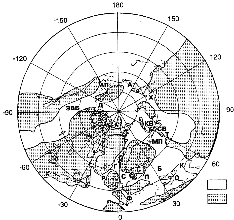
Рис. 1. Схема расположения проливов Северного полушария: МП — Мезенско-Печорский пролив, К — Каспийский пролив, О — Ореховский проход, КВ — Карские Ворота, СВ — Сосьвинские Ворота, Т — Туринский пролив, Б — Брестский пролив, Г — Гренландский пролив, Р — пролив Роколл, Ф — Французский пролив, П — Польский пролив, С — Североморский пролив, А — Анжуйский пролив, Х — Хатангский проход, Д — пролив Доусон, АП — Аляскинский пролив, ЗВБ — пролив Западного Внутреннего бассейна; 1 — море; 2 — суша
